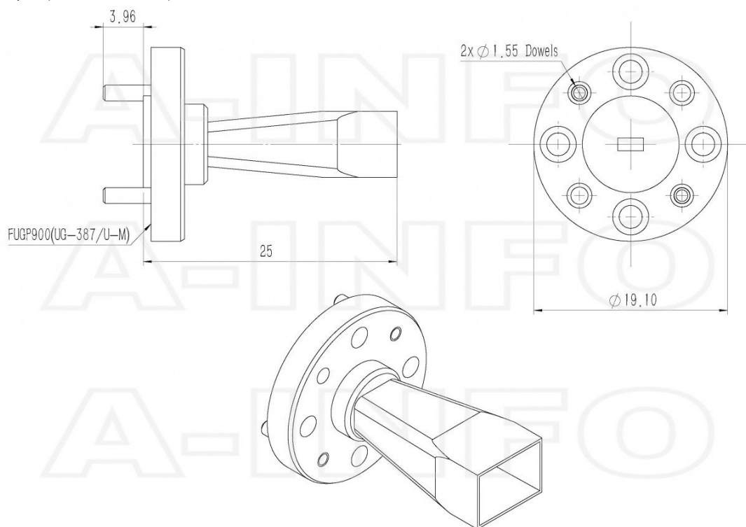
FUGP900 Output (P/N: LB-10-15-A)
